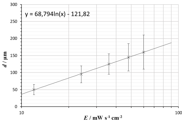
Abbildung 1: Arbeitskurve von SKresin 1335 – NEON gelb
