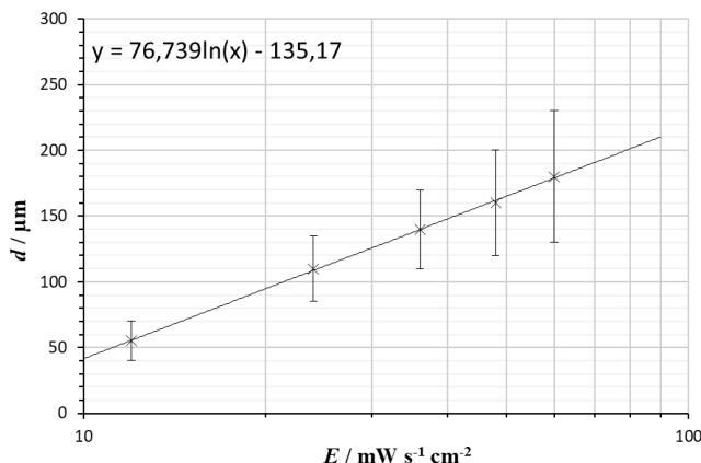
Abbildung 3: Arbeitskurve 1335 – NEON orange
