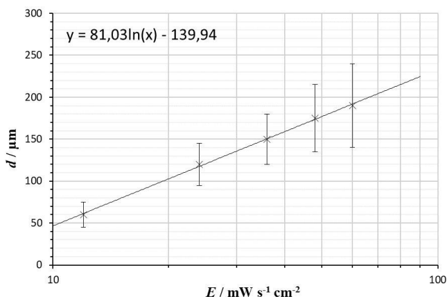
Abbildung 4: Arbeitskurve 1335 – NEON pink.
