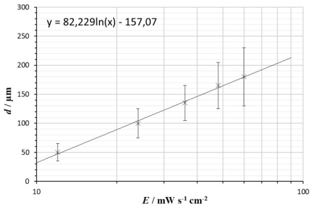
Abbildung 2: Arbeitskurve von SKresin 1335 – NEON grün
