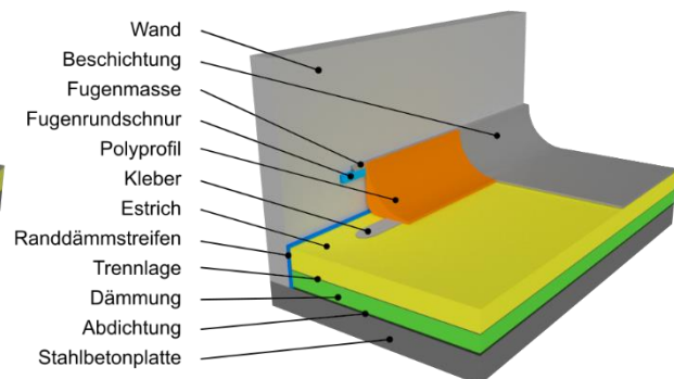
POLYPROFIL® - Hohlkehlen 5/5 auf einem schwimmenden Estrich
