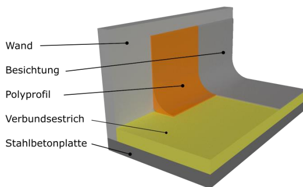
POLYPROFIL® - Hohlkehlen 2.5/10 auf einem Verbundestrich
